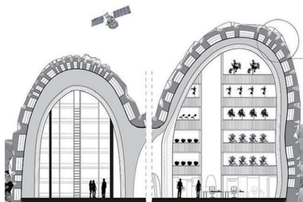
图5 “Test Lab”结构的纵向剖面
